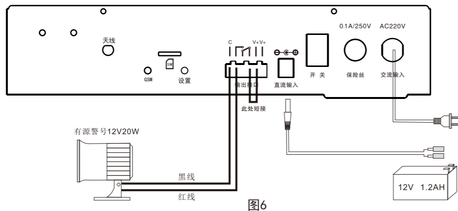
KS-600C报警主机的系统连接(如图6)
