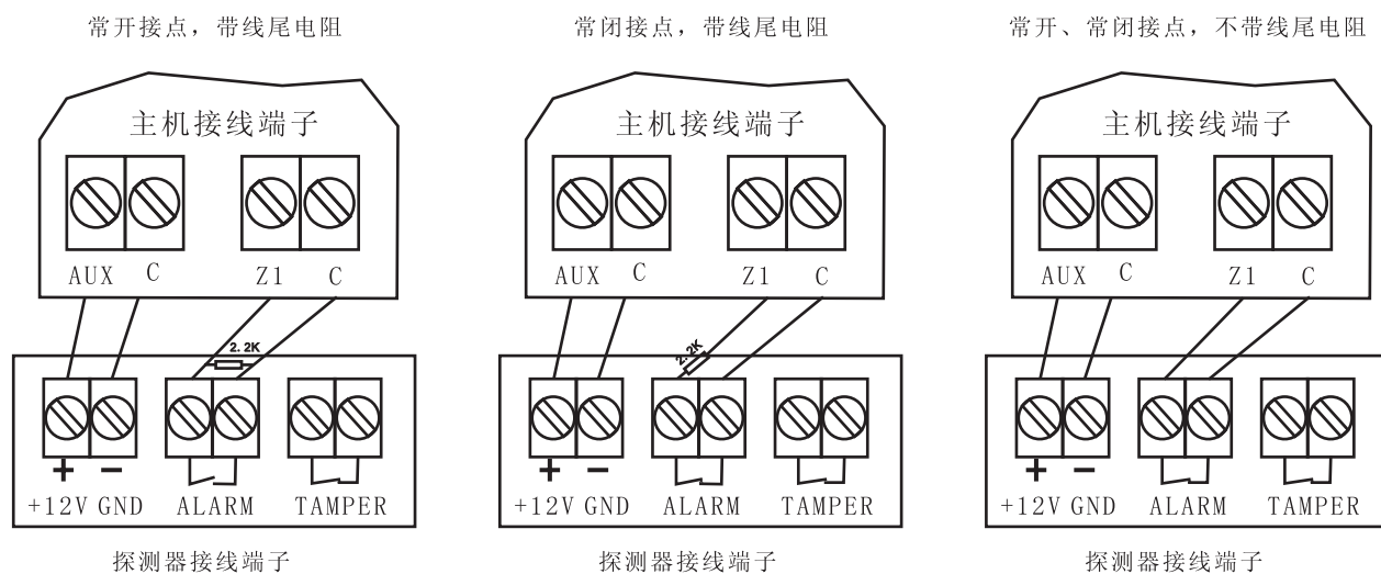
图二 有线防区接线图
