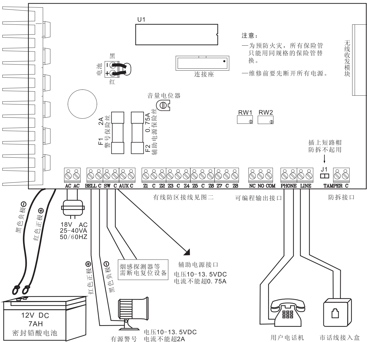
图一 主机接线图
